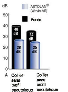
L'influence du caoutchouc au niveau du bruit A: Rapport des Institut für Schall- und Wärmeschutz Prof. Dr. Zeller, Essen. Rapport d'essai: 15.216 Le rapport peut être obtenu chez Wavin. Le poids de surface de la cloison: 80 kg/m²
